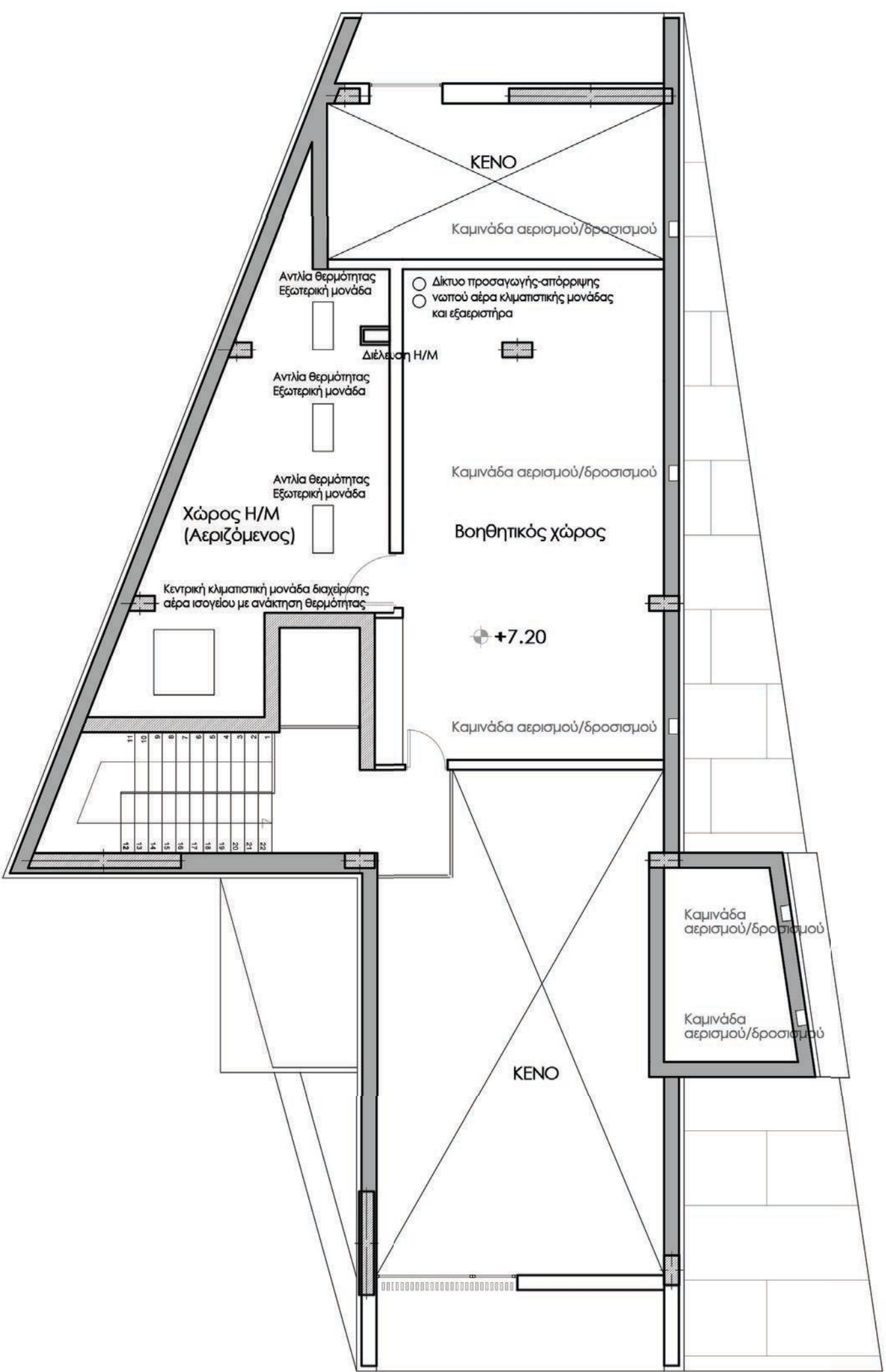
ΚΑΤΟΨΗ ΠΑΤΑΡΙΟΥ ΚΛ.1/100
