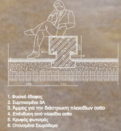
ΓΡΑΜΜΙΚΟ ΚΑΘΙΣΤΙΚΟ ΤΟΜΗ 1/20
