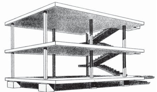
L'ossature standard « Dom-ino », pour exécution en grande série
